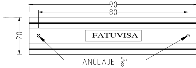
VISTA PLANTA
