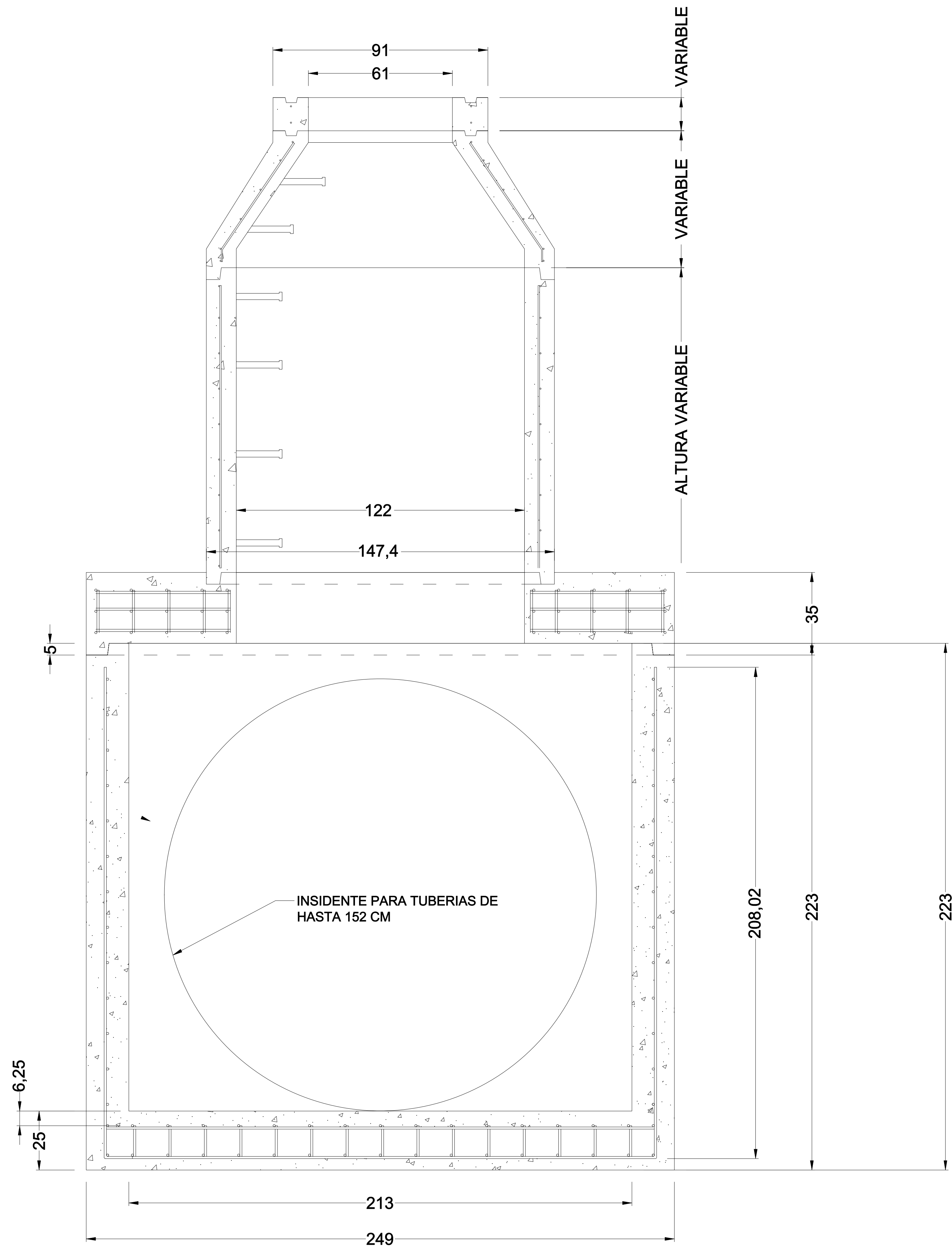
2 DETALLES DE POZO TIPO CAJA COMPLETO
